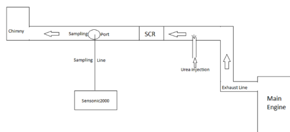
Fig. 13 SCR rig
