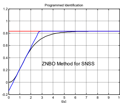
(d) ZNOL for SNSS
